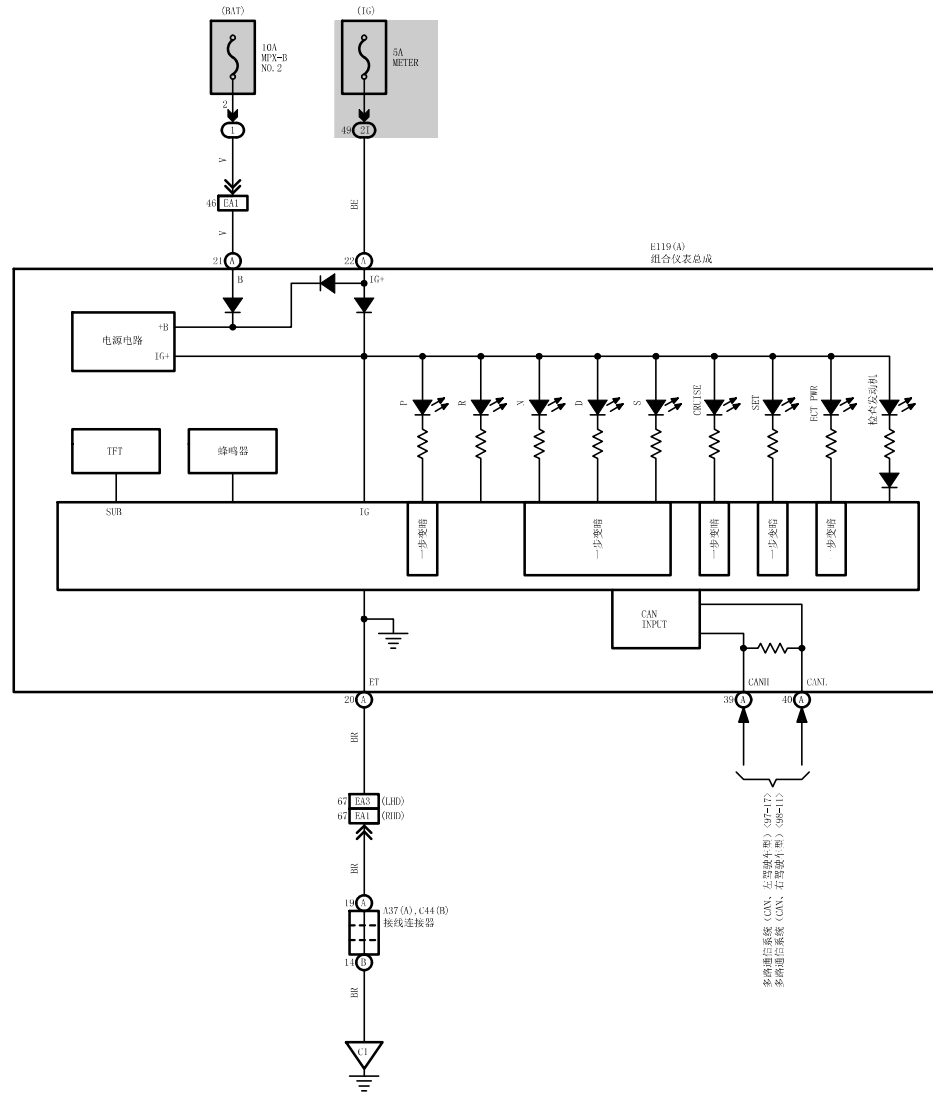
ECT 和 A/T 档位指示器 (1GR-FE) (2015 年 8 月之后生产)
